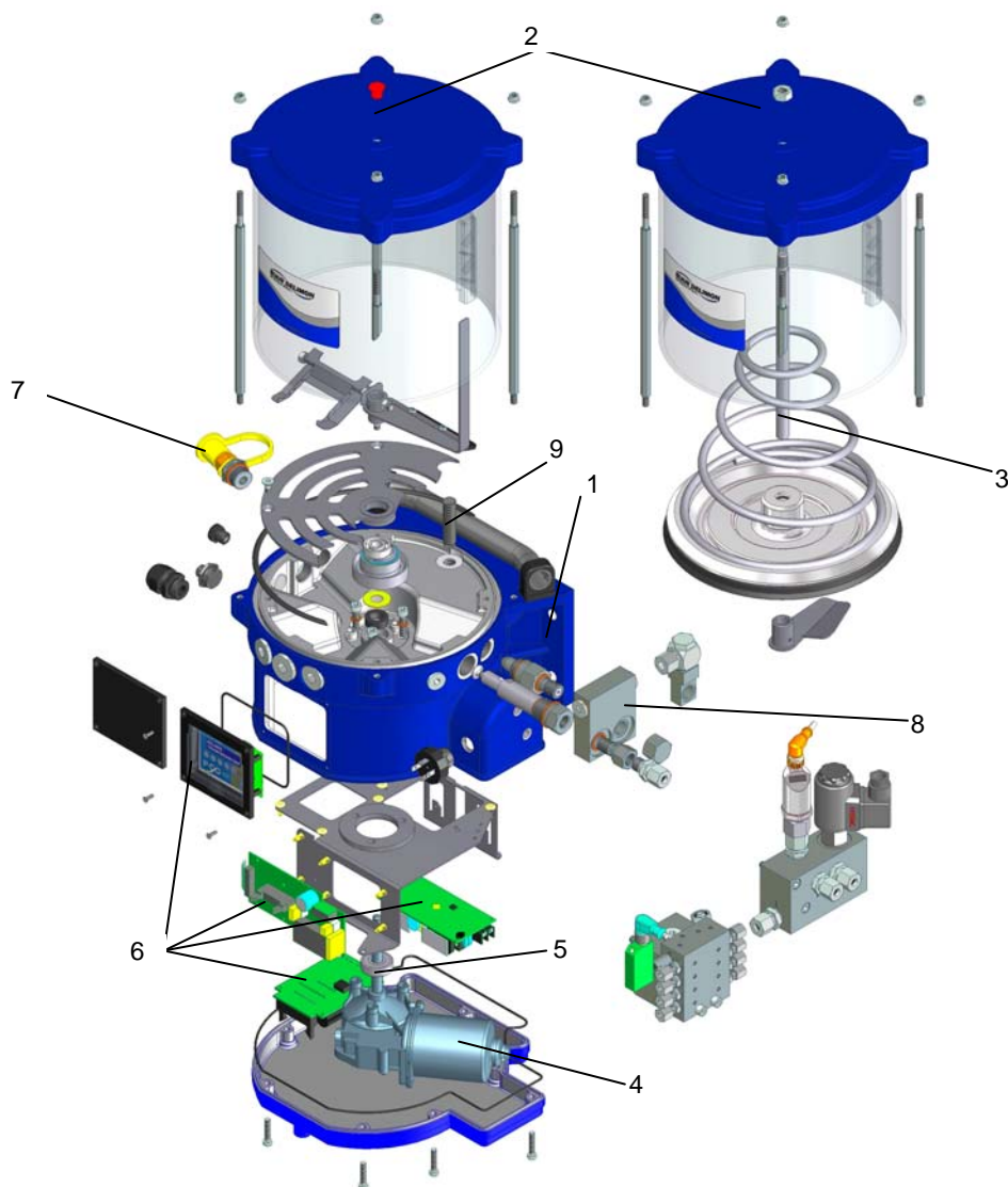
Fig 1 (Pump design)
